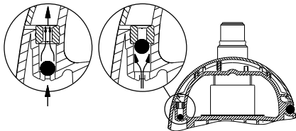
Fig. 12 Purge
